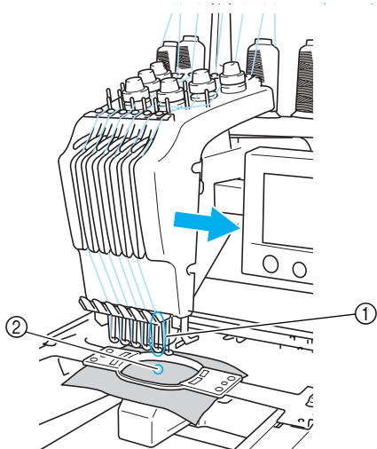
① Игла в позиции вышивки Игла размещается над отверстием в игольной пластине ②.
