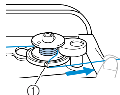
① Прорезь в седле намотки шпульки (со встроенным устройством обрезки)
