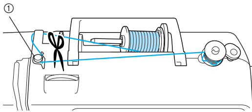
1 Нитенаправитель для намотки катушки
