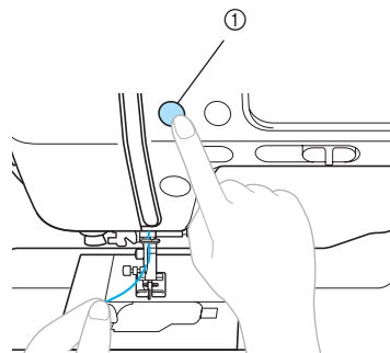
① Кнопка позиционирования иглы
