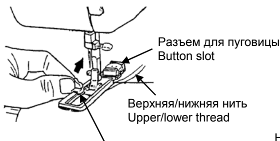
Приспособление для установки пуговицы Button adjuster
